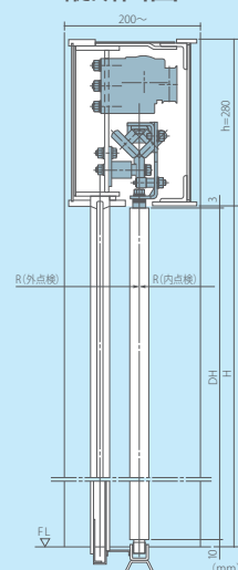
縦断面図
