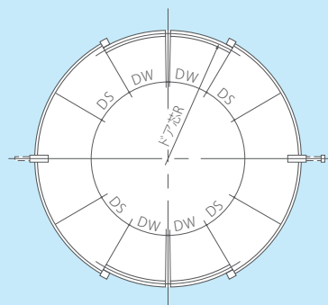
平面図(円形引き戸)
